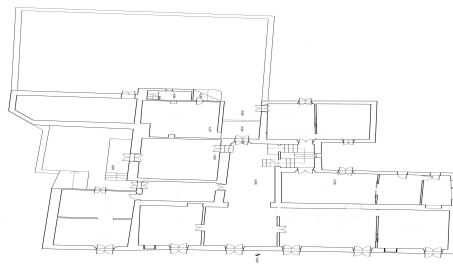
Planta 1ª
